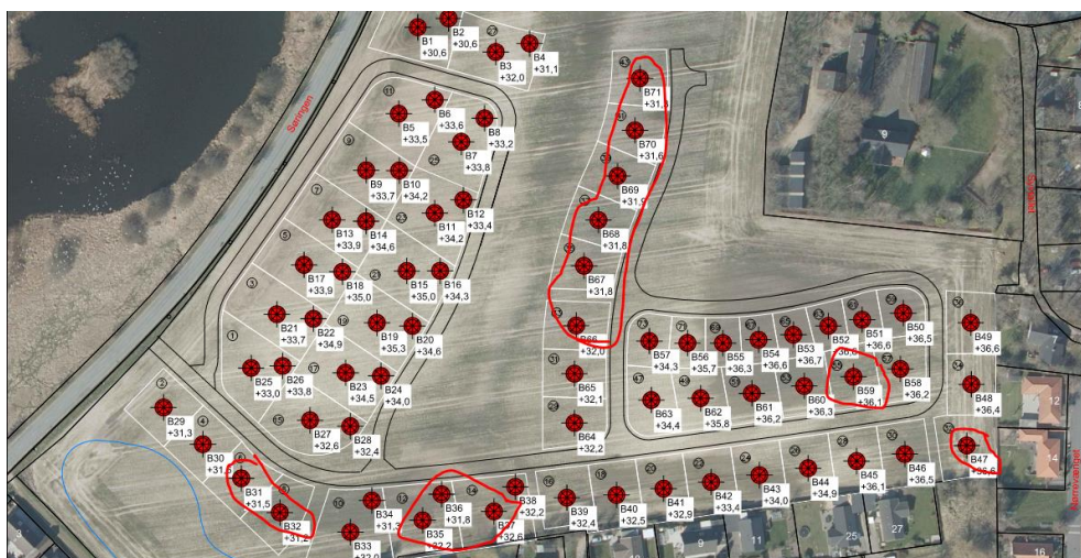
Figur 3 Placering af boringer på projektområdet. I boringer markeret med rød cirkel er der konstateret sande aflejringer i et sådant omfang, at der sandsynligvis skal etableres sugespidsler til håndtering af grundvand.
